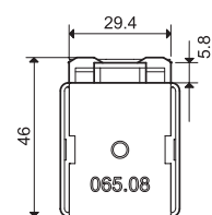
Adaptador con aletas en carril 35 mm (EN 60715) en la parte posterior para tipos 65.31.x.xxx.xxx9
