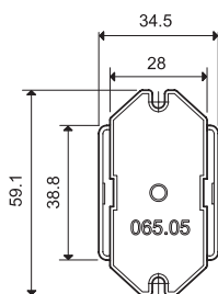
Adaptador con aletas de sujeción frontal para tipos 65.31.x.xxx.xxx9
