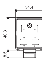
Adaptador con aletas en carril 35 mm (EN 60715) en la parte superior para tipos 65.31.x.xxx.xxx9
